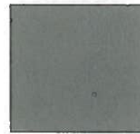
49 Gray PAS6-C0001
